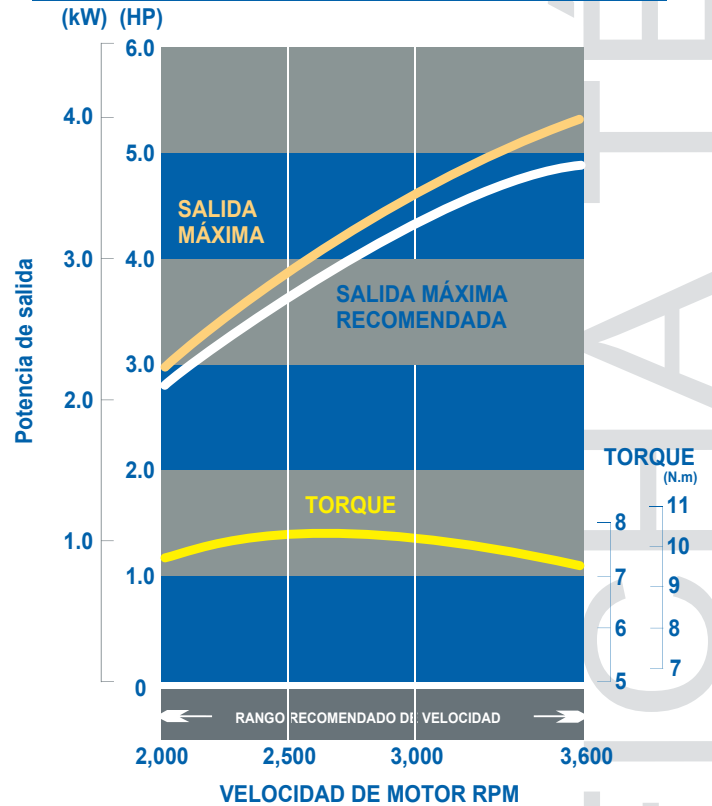
CURVA DE DESEMPEÑO MP-5.5
