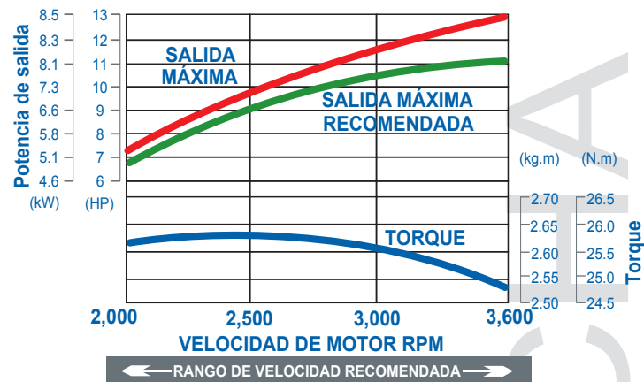
CURVA DE DESEMPEÑO
